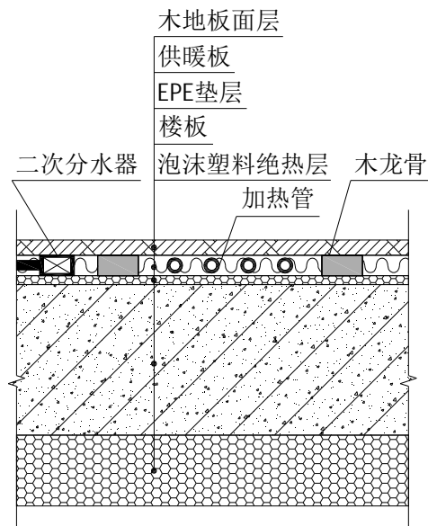
图 A. 3. 4 预制轻薄供暖板地面构造 (四) 注: 与室外空气或不供暖房间相邻、以木地板面层为例
