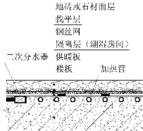
图 A. 3. 3 预制轻薄供暖板地面构造 (三) 注: 与供暖房间相邻、潮湿房间
