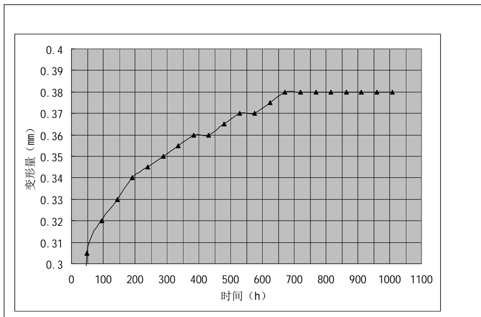
图 4 预制轻薄供暖板长期局部荷载试验结果
