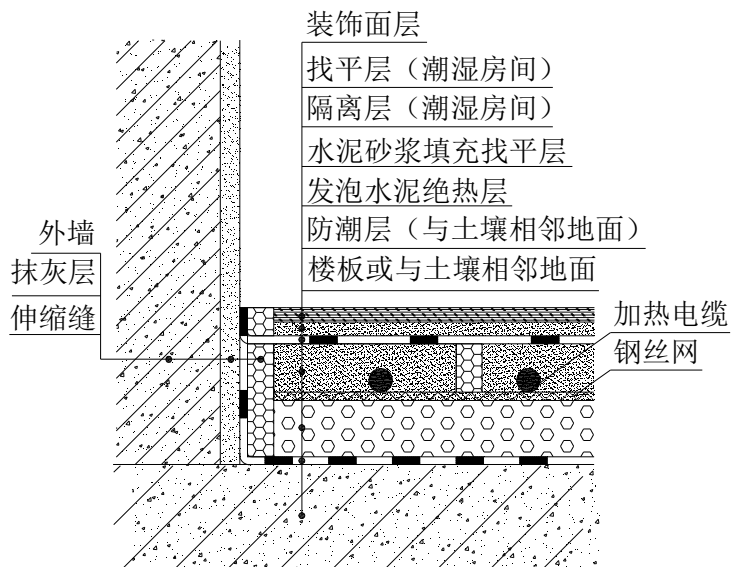
图 A.1.4 混凝土填充式加热电缆供暖地面构造 (二) 注: 采用发泡水泥绝热层
