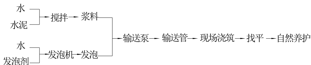
图5.2.3-1 物理发泡工艺图
