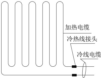
图 F.2.1 单导加热电缆单路平行布置
