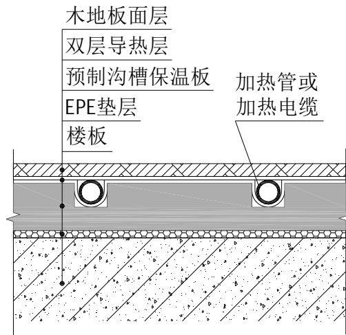
图 A.2.1 预制沟槽保温板供暖地面构造（一）
