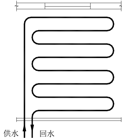
图 F.1.2 平行型布置
