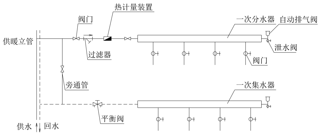
图 E. 1. 1 直接供暖系统示意图
