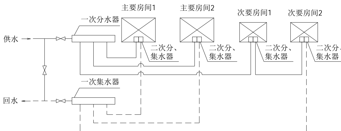
图 D.0.4 预制轻薄保温板地面供暖系统示意
