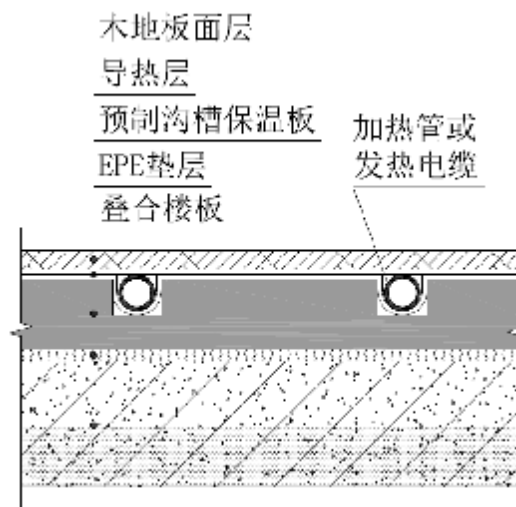
图 A. 2. 6 预制沟槽保温板供暖地面构造（六）
