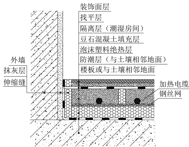
图 A.1.3 混凝土填充式加热电缆供暖地面构造 (一) 注: 采用泡沫塑料绝热层
