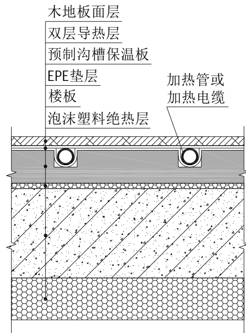
图 A.2.2 预制沟槽保温板供暖地面构造（二）
