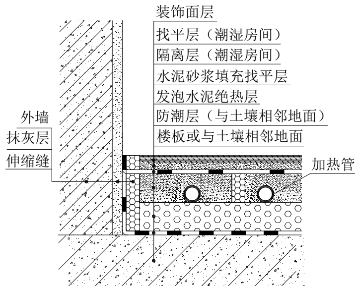
图 A.1.2 混凝土填充式热水供暖地面构造 (二)
