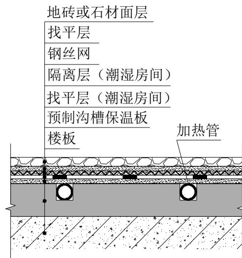
图 A.2.4 预制沟槽保温板热水供暖地面构造（四） 注：与供暖房间相邻、地砖或石材面层
