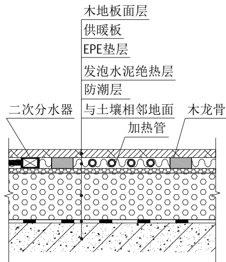
图 A.3.5 预制轻薄供暖板地面构造（五）
