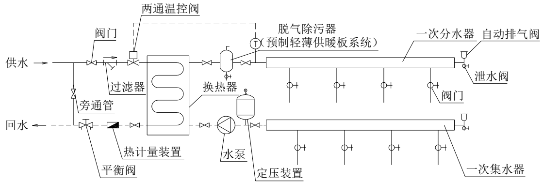
图 E.2.1 间接供暖系统示意图
