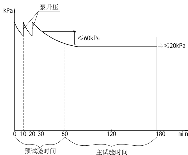
图 6.4.3 水压试验时间分配和压力示意
