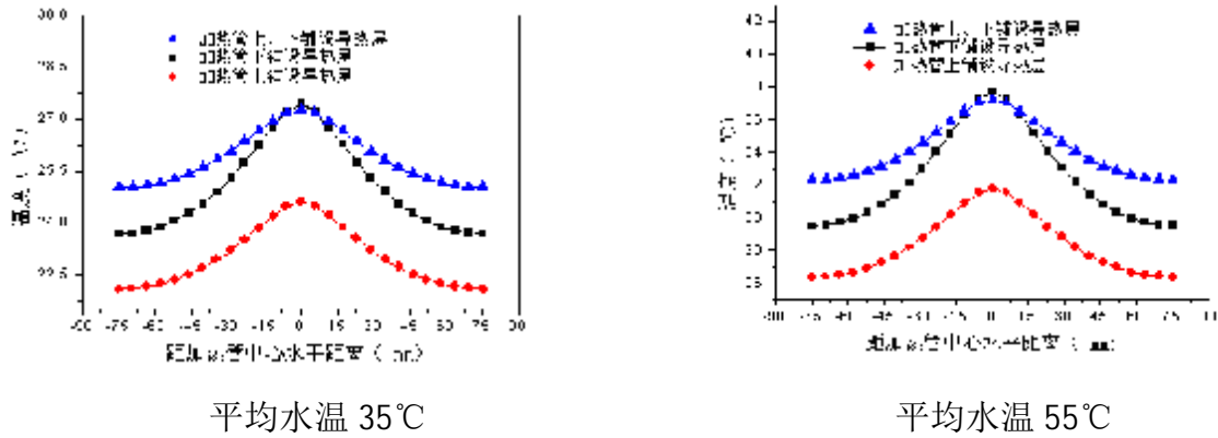
图 2 导热层铺设在不同位置时地面温度分布
