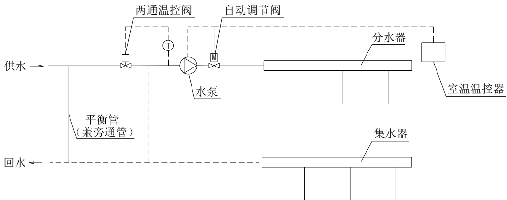
图 J.0.3 混水系统分户控温示意图
