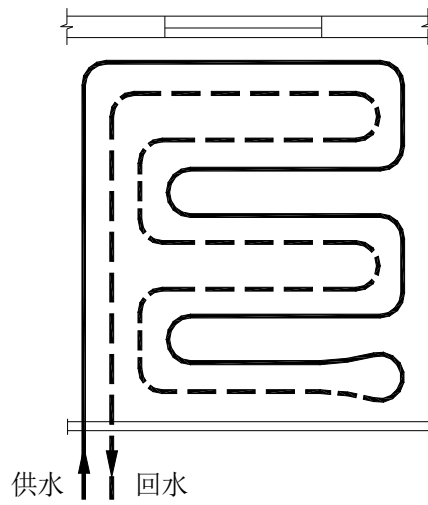
图 F.1.3 双平行布置
