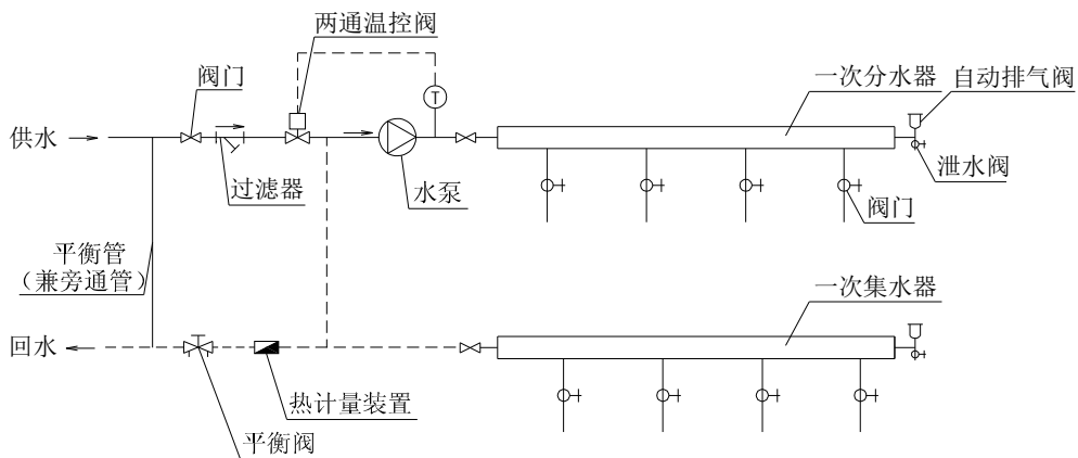
图 E.3.2 采用两通阀的混水系统
