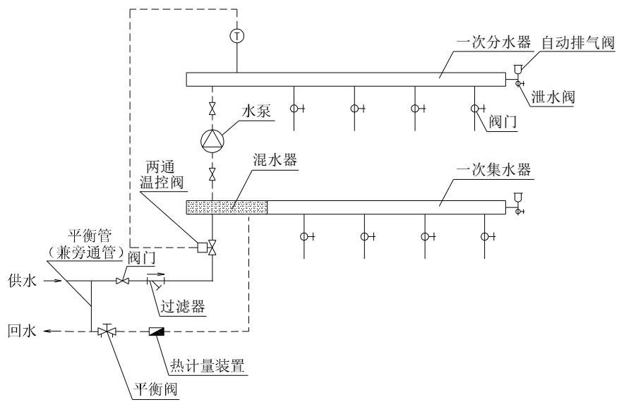
图 E.3.3 设置混水器的系统
