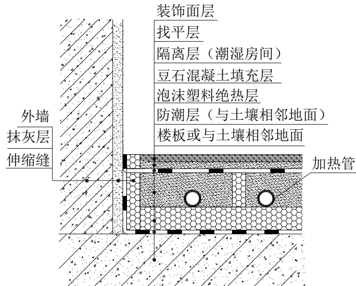
图 A.1.1 混凝土填充式热水供暖地面构造 (一)
