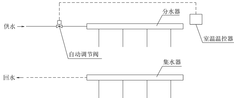
图 J.0.1 总体（分户）控温示意图
