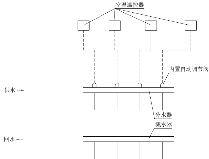
图 J.0.2 分环路（分室）控温示意图
