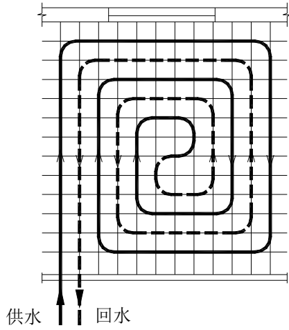
图 F.1.1 回折型布置
