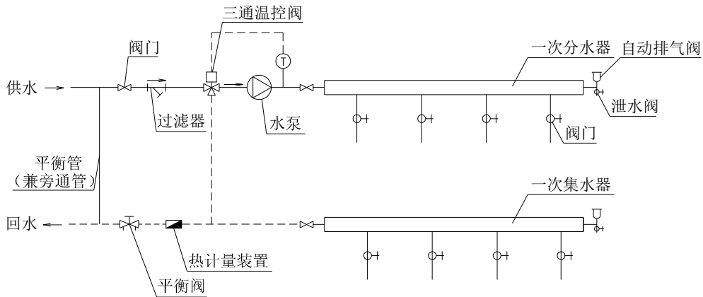
图 E.3.1 采用三通阀的混水系统
