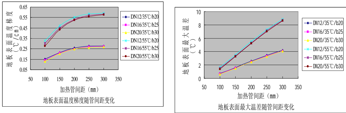
图5 不同管间距地板表面的温度梯度和最大温差
