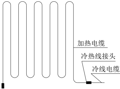
图 F.2.2 双导加热电缆平行布置
