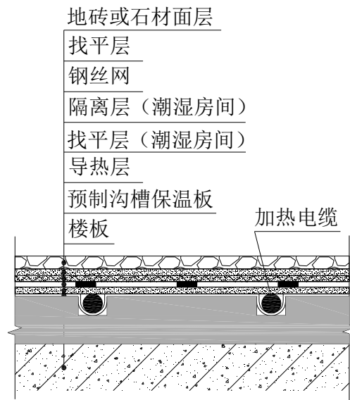
图 A. 2. 5 预制沟槽保温板加热电缆供暖地面构造（五）
