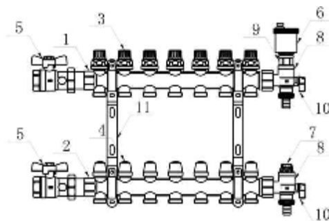
图6 分水器集水器装置结构图
