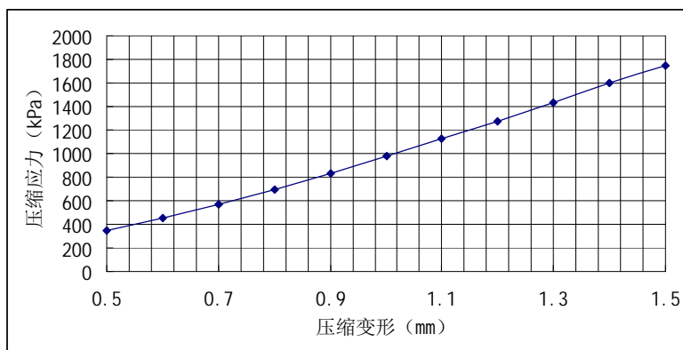
图5 预制沟槽保温板供暖地面试件短期局部荷载试验结果
