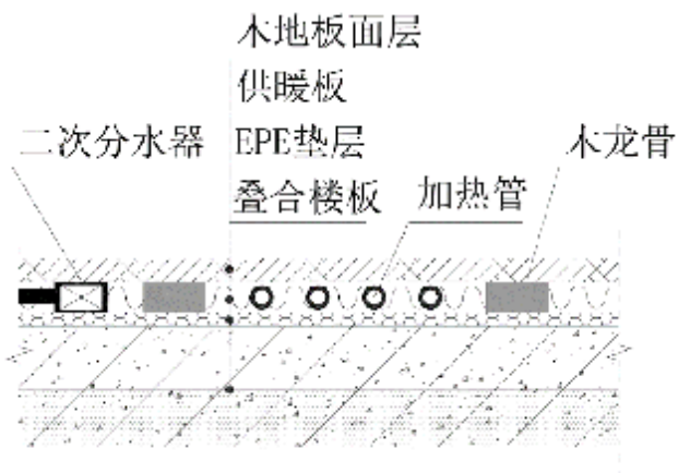
图 A.3.6 预制轻薄供暖板地面构造（六）
