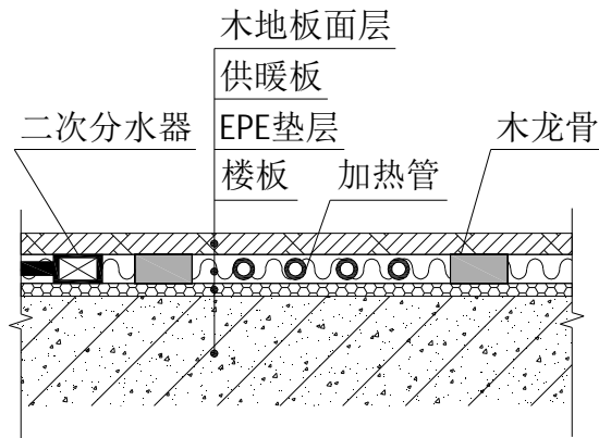
图 A.3.1 预制轻薄供暖板地面构造示意（一）
