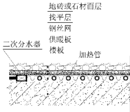
图 A.3.2 预制轻薄供暖板地面构造（二）
