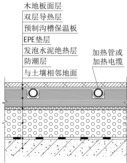
图 A.2.3 预制沟槽保温板供暖地面构造（三） 注：与土壤相邻、以木地板面层为例
