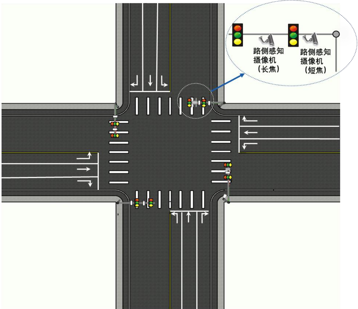
图 A.2 十字路口利旧设备布设示意图
